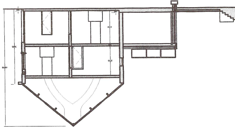
Doorsnede AA' gewijzigd 1/200
